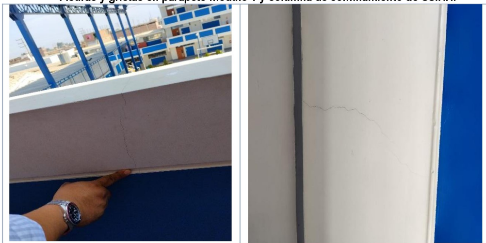
Imágenes n.º 8 y 9 Fisuras y grietas en parapeto modulo 1 y columna de confinamiento de SS.HH.
