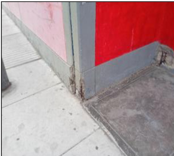
Cerco perimétrico de la puerta de ingreso de la I.E. 88024 presenta desprendimiento de concreto.
