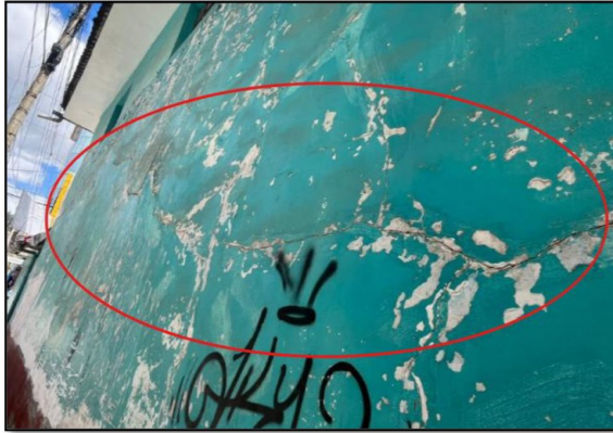
Fisuras Horizontales y pérdida de capa de pintura en el muro perimétrico – I.E 86017 Sabio Antonio Raimondi
