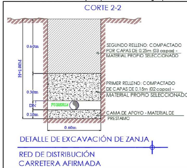
Imagen n.° 1 Relleno a nivel de la calzada y compactada en red de agua potable
