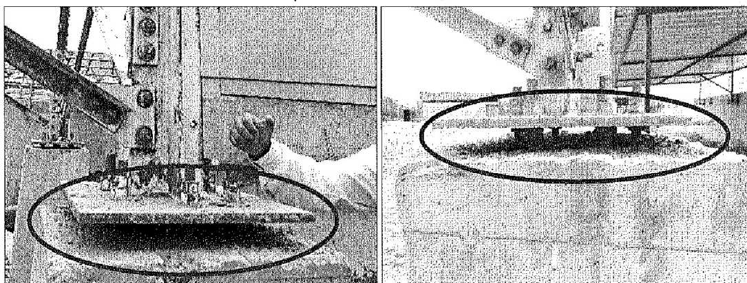
Imágenes n.ºs 38 y 39 Pernos de anclaje no embebidos en pedestal de concreto
