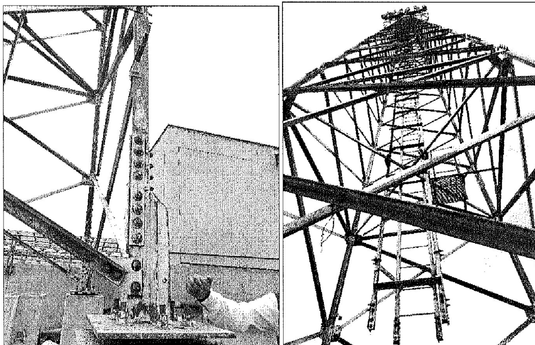
Imágenes n.ºs 28 y 29 Desgaste de pintura, oxidación y corrosión en torre de iluminación (Nor – este)
