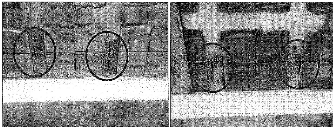
Imágenes n.ºs 18 y 19 Cangrejas con refuerzo de acero expuesto y con presencia de oxidación en losas aligeradas
