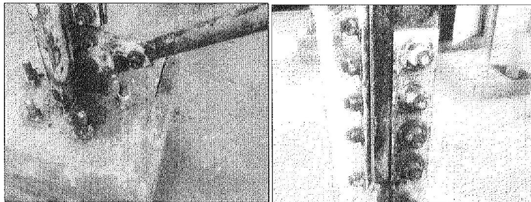
Imágenes n.ºs 30 y 31 Desgaste de pintura, oxidación y corrosión en torre de iluminación (Nor – oeste)
