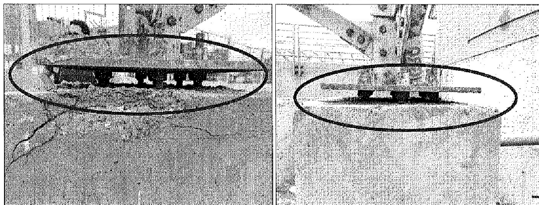
Imágenes n.ºs 36 y 37 Pernos de anclaje no embebidos en pedestal de concreto
