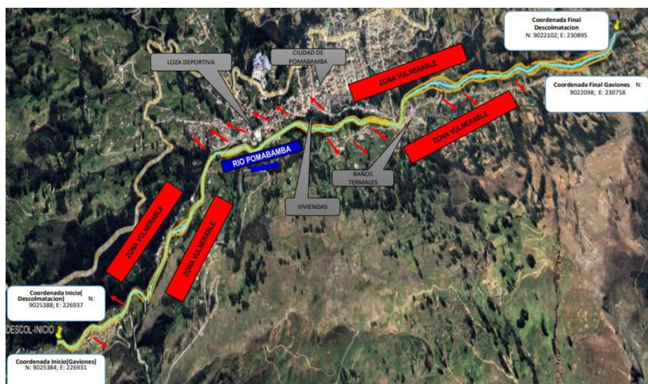
IMAGEN N° 3 IMAGEN SATELITAL DE LA ZONA VULNERABLE – RIO POMABAMBA
