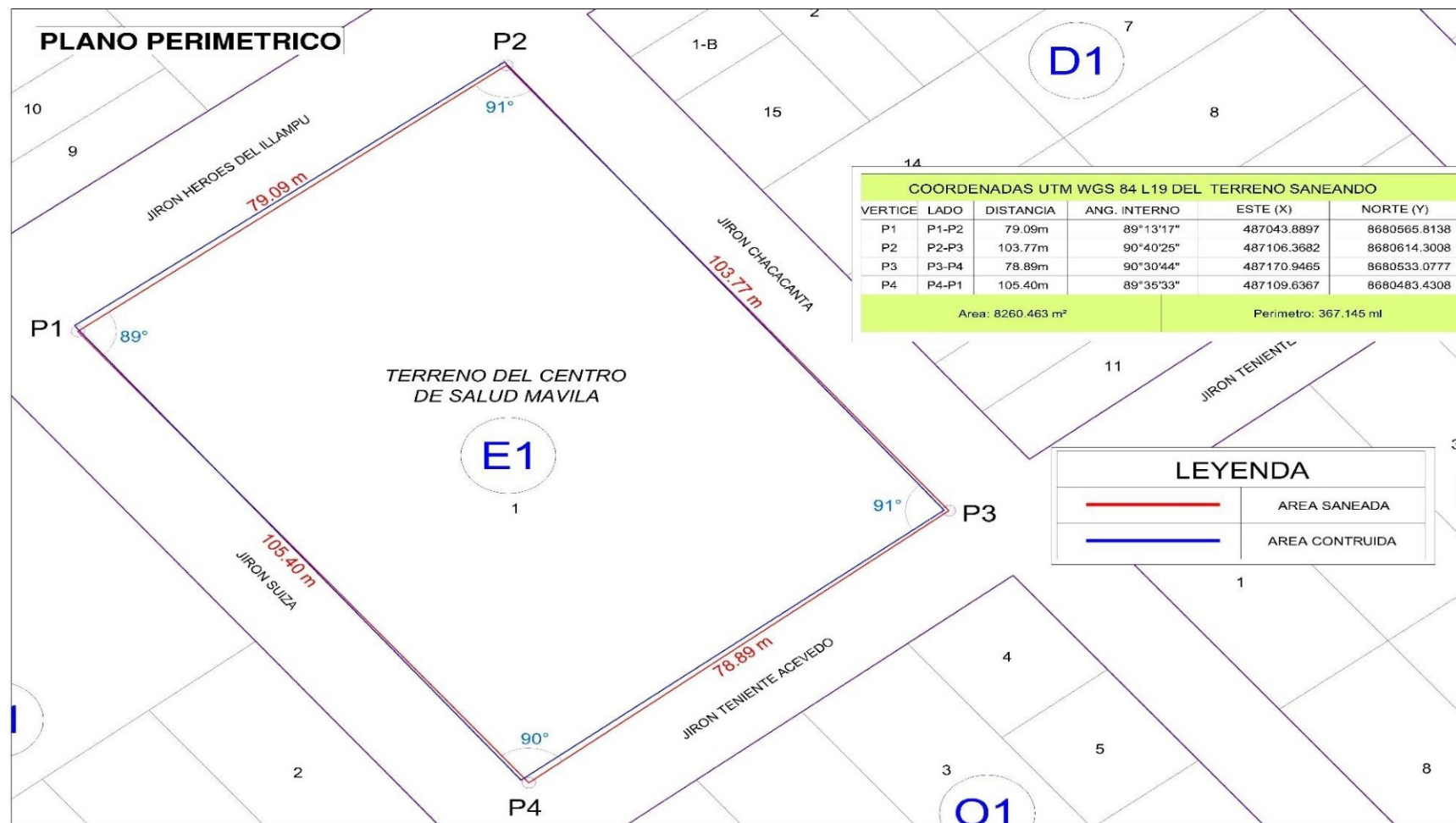
Imagen n.º 14 Plano perimétrico del área saneada y área construida
