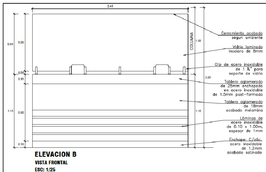
Imagen n.º 1 Vista frontal como correspondería culminar los trabajos y materiales a utilizar
