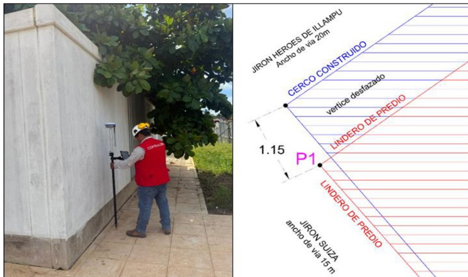
Imagen n.° 15 Verificación del vértice P1
