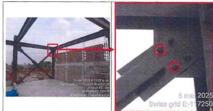
En la unión de la conexión de esquina de la diagonal del arriostre metálico, se evidencia perforaciones circulares próximos a los pernos atornillados
