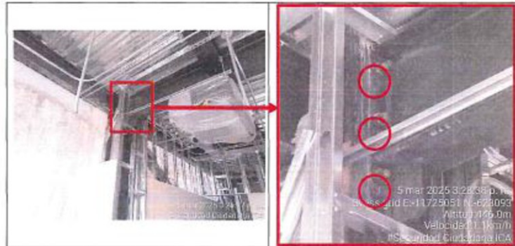
Unión de viga-columna de la estructura metálica del primer nivel, presenta perforaciones circulares próximas a los pernos atornillados, se percibe que fueron rellenos con una parte metálica sin soldar
