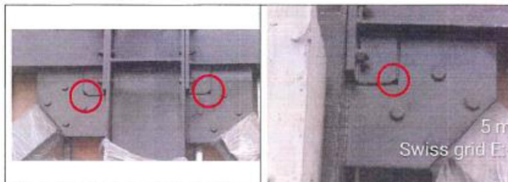
Aberturas en las uniones de la parte soldada en conexiones de esquina de diagonales de arriostres metálicos
