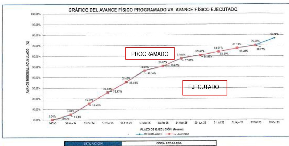
Imagen n.º 5 Gráfico de Curva "S"
