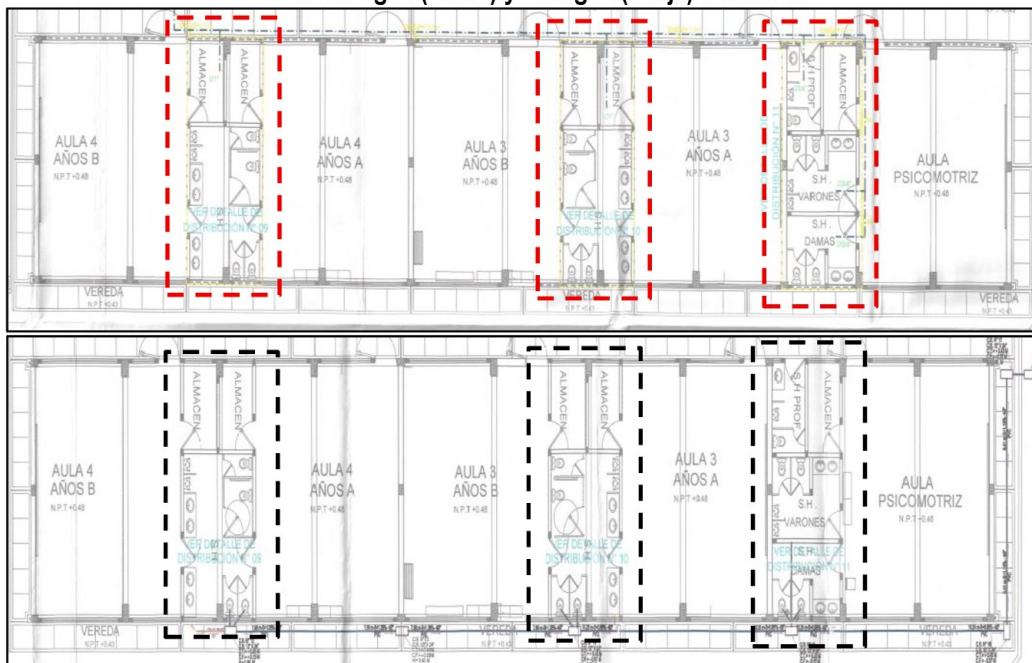
Imagen n.° 18 Red de Agua (Arriba) y Desagüe (Abajo) Modulo IX
