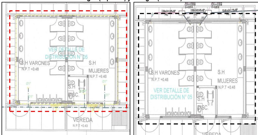
Imagen n.º 14 Red de Agua (Izquierda) y Desagüe (Derecha) Modulo VI
