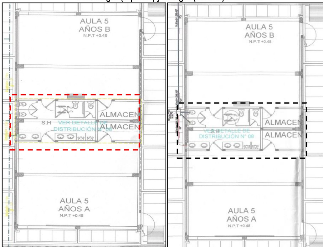
Imagen n.º 17 Red de Agua (Izquierda) y Desagüe (Derecha) Modulo VIII
