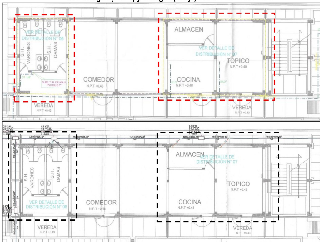
Imagen n.º 15 Red de Agua (Arriba) y Desagüe (Abajo) Modulo VII – 1ER PISO
