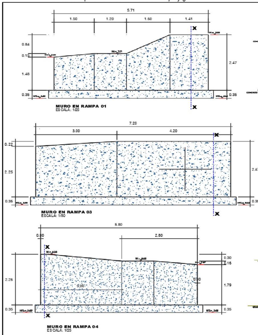
Imagen n.º 8 Detalle del plano “DRG-02-Detalle de rampa y gradería 01”
