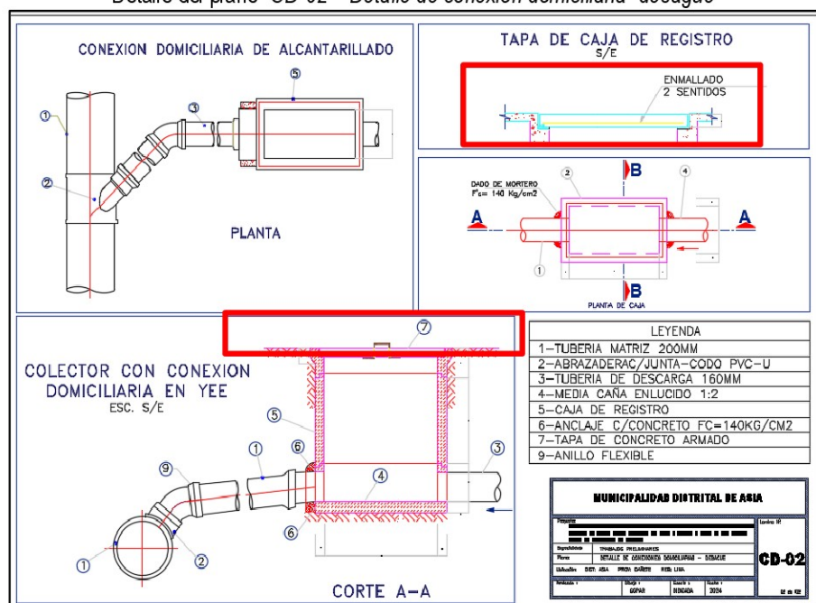
Imagen n.º 6 Detalle del plano "CD-02 – Detalle de conexión domiciliar-desagüe"
