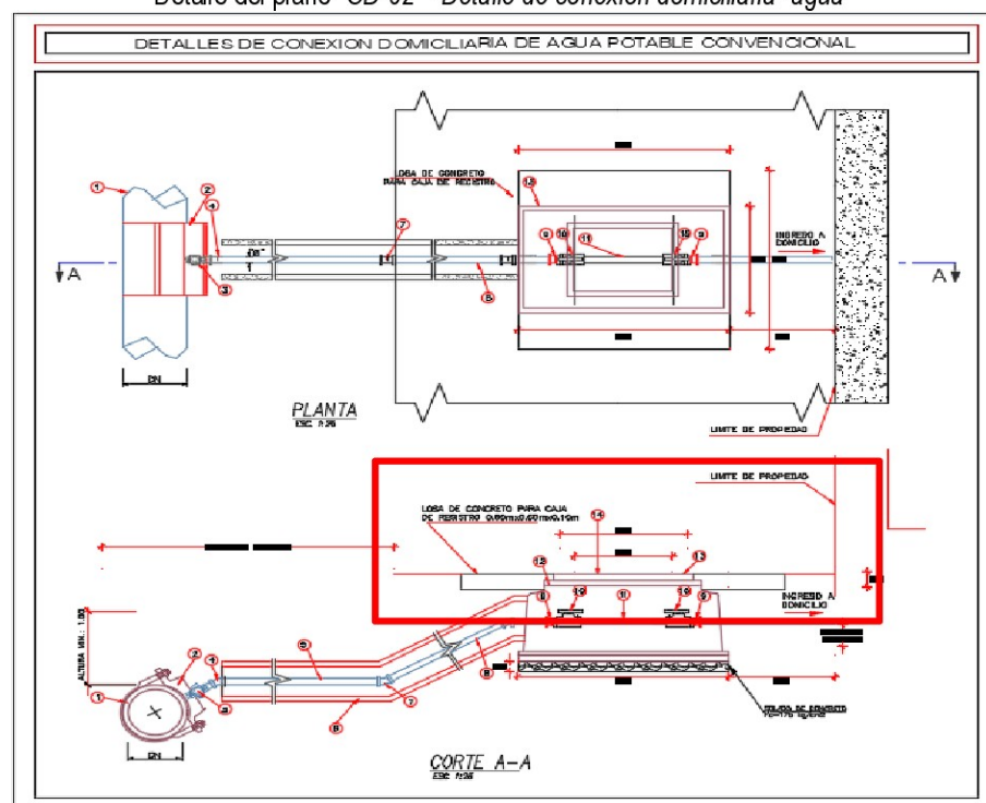
Imagen n.º 7 Detalle del plano "CD-02 – Detalle de conexión domiciliar-agua"
