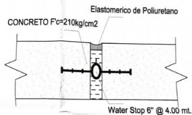
DETALLE DE WATER STOP ESCALA 1:10
