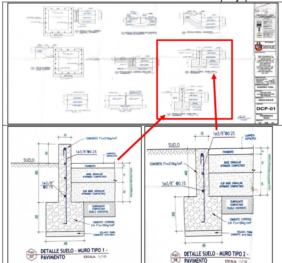
Imagen n.° 98 Plano DCP-01 indica diseño de los muros de sostenimiento tipo 1 y tipo 2.
