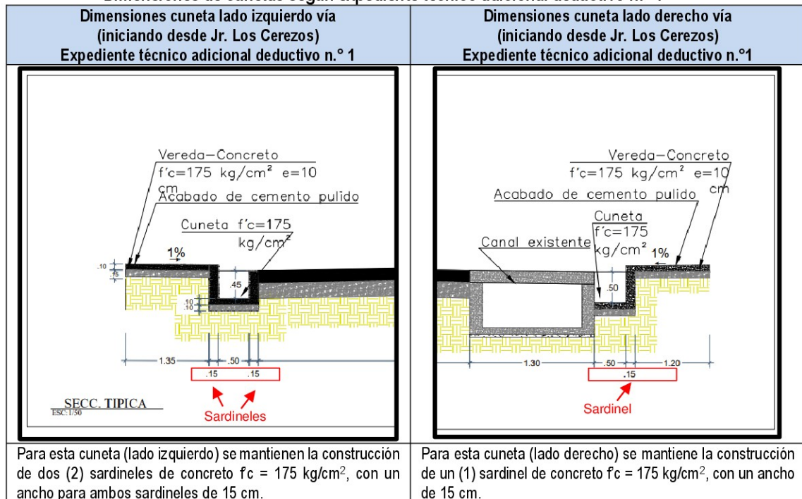
Figura n.º 2 Dimensiones de cunetas según expediente técnico adicional deductivo n.º 1
