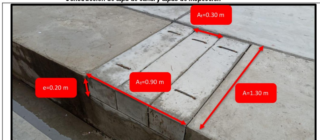
Fotografía n.º 14: Se verifica la construcción de la tapa de canal de concreto y tapas de inspección.
