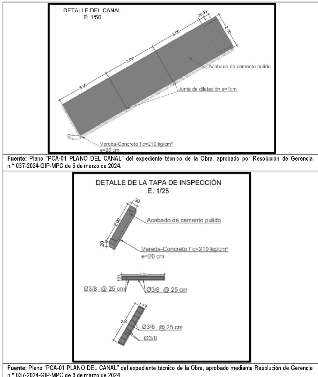
Figura n.º 5 PCA-01 PLANO DEL CANAL
