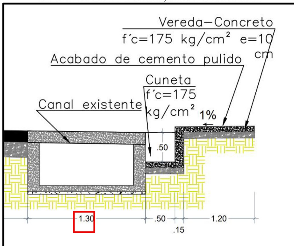
Figura n.º 7 PLANO ST-01 DETALLE DE JUNTAS, PAÑOS Y SECCIÓN TÍPICA
