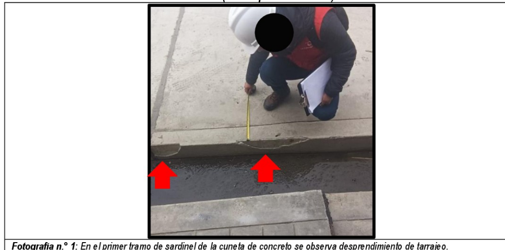
Fotografías n.ºs 1 a 10 Sardinel en cuneta (lado izquierdo de la vía)
