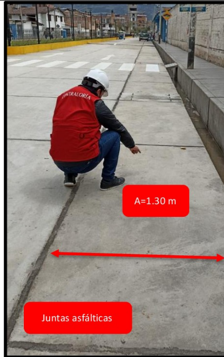
Fotografía n.º 16: Se observa la tapa de concreto de canal, al lado derecho de la vía, la cual posee un ancho de 1.30 m. y cuenta con tapas de inspección.
