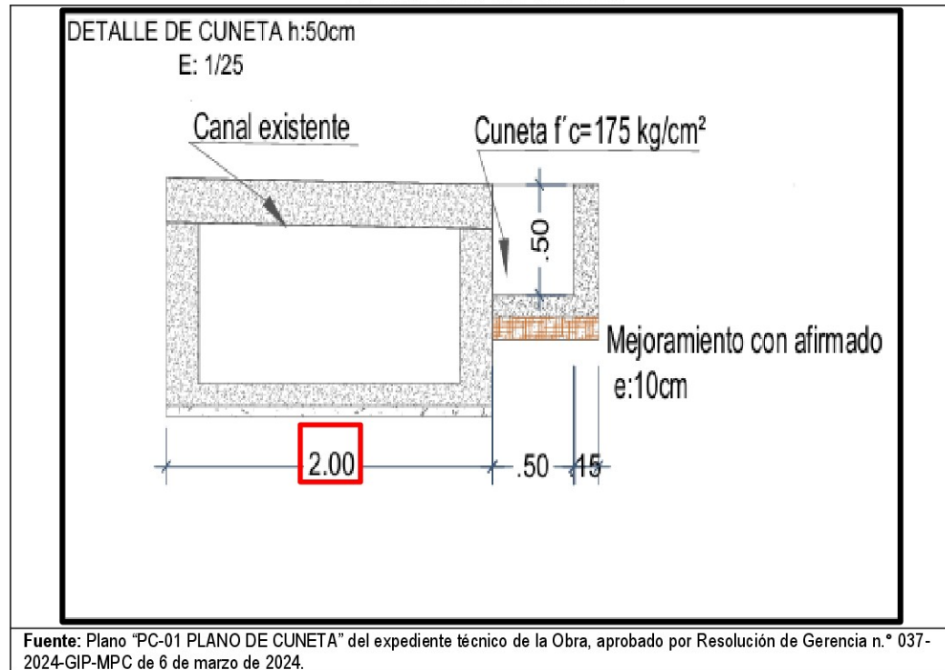
Figura n.º 6 PC-01 PLANO DE CUNETA
