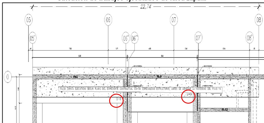
Imagen N° 9 Ubicación de trabajos ejecutados de falsa zapata
