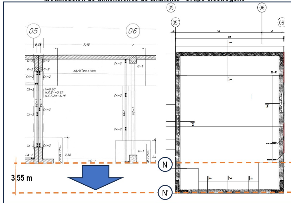
Imagen N° 8 Modificación de dimensiones de ambiente "Grupo electrógeno"
