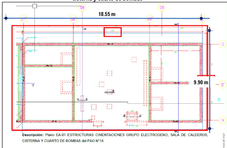
Imagen N° 6 Plano EA-01 "Estructuras cimentaciones grupo electrógeno, sala de calderos, cisterna y cuarto de bombas"
