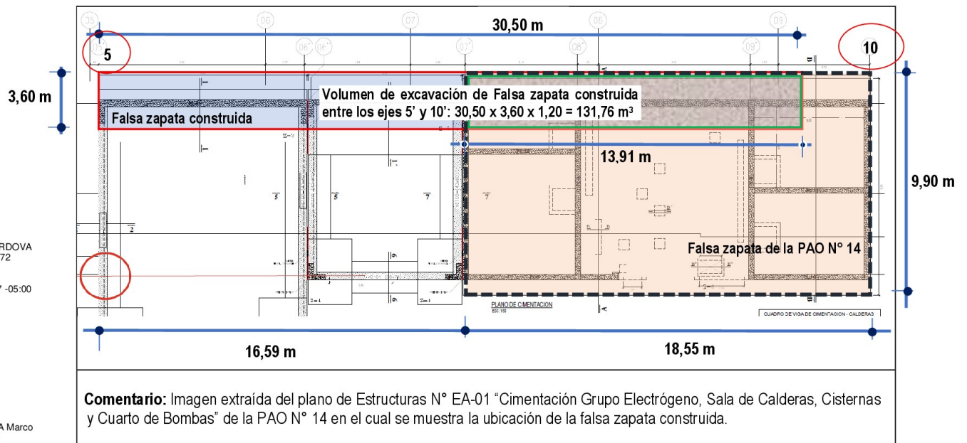
Imagen N° 11 Ubicación de trabajos de excavación ejecutados de falsa zapata entre los ejes 5' y 10'
