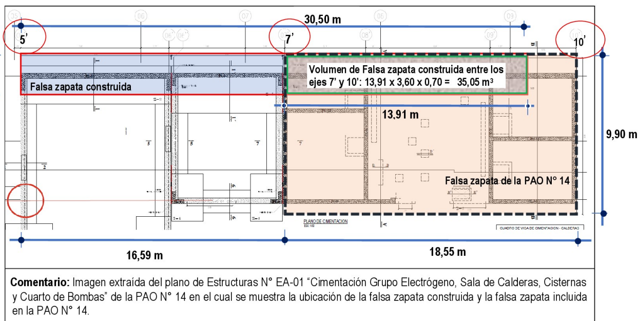
Imagen N° 7 Ubicación de trabajos ejecutados de falsa zapata entre los ejes 5' y 10'
