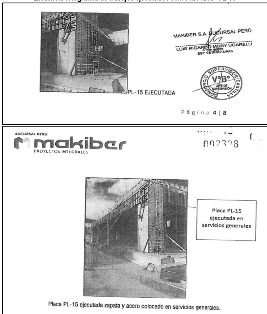
Imagen N° 3 Evidencia fotográfica de trabajos ejecutados sobre la Placa “PL-15”
