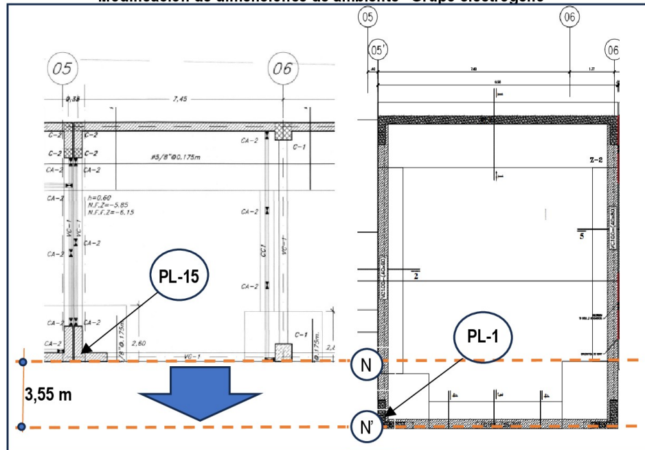
Imagen N° 5 Modificación de dimensiones de ambiente "Grupo electrógeno"
