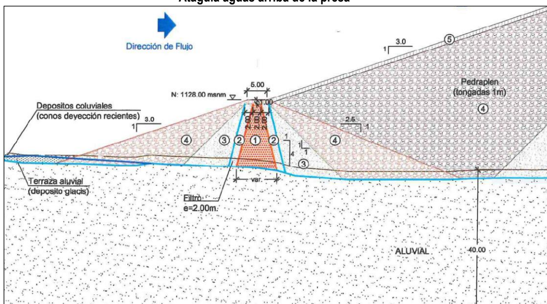
Imagen N° 3 Ataguía aguas arriba de la presa
