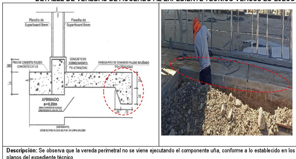
IMAGEN N° 6 DETALLE DE VEREDAS DE ACUERDO AL EXPEDIENTE TÉCNICO VERSUS LO EJECUTADO
