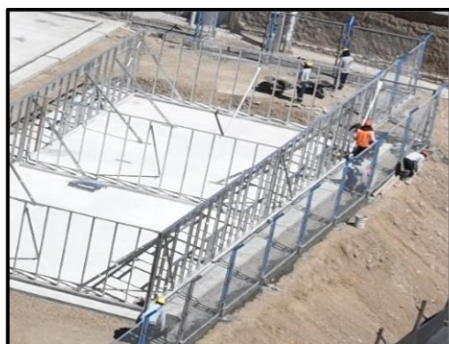
IMAGEN N° 10 VISTA DE LAS CIMENTACIONES DEL CERCO PERIMÉTRICO DE MALLA OLÍMPICA, EL CUAL SE HA CIMENTADO SOBRE MATERIAL DE RELLENO MUY CERCANO AL TALUD, SIN TRATAMIENTO PREVIO
