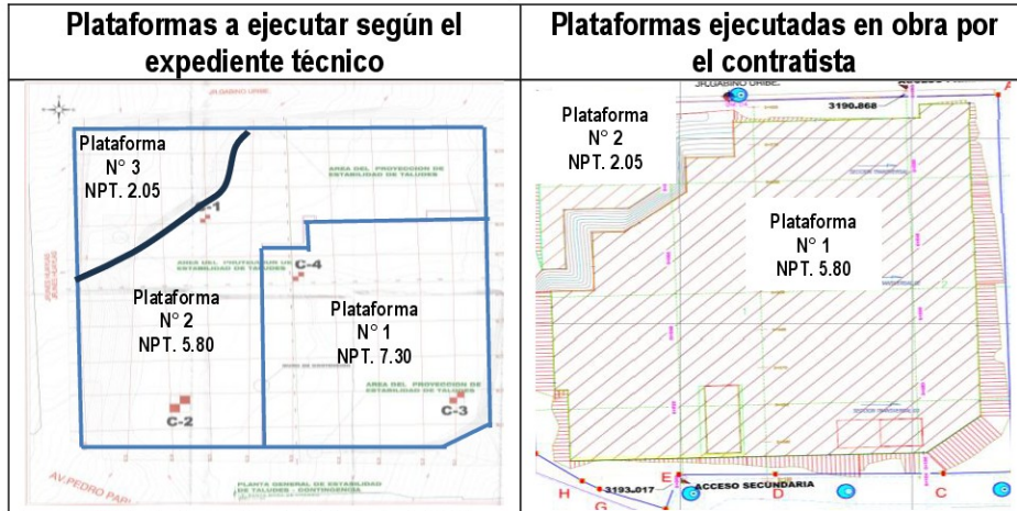
IMAGEN N° 12 VISTA DE PLATAFORMAS REQUERIDAS VS EJECUTADAS
