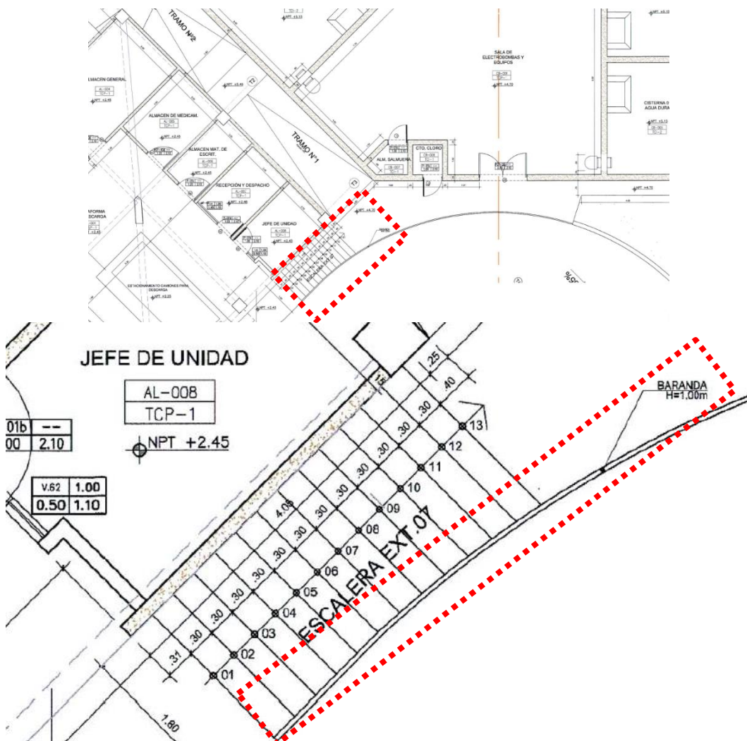
Imagen N° 02: Plano de arquitectura A-30- Detalle de escalera 8 que da acceso al área de cisternas
