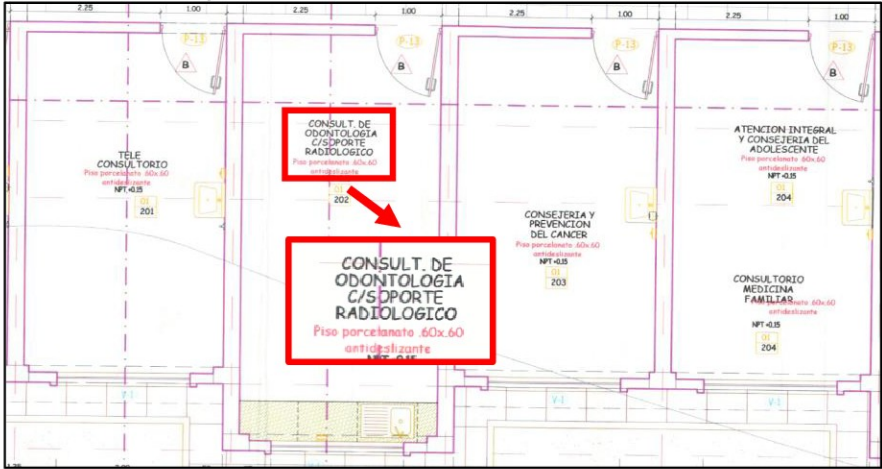
Imagen n.º 25 Piso porcelanato antideslizante en ambientes interiores
