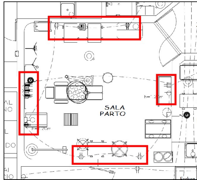
Imagen n.º 21 Tomacorrientes ubicados en muros en Sala de Partos según plano IE-16
