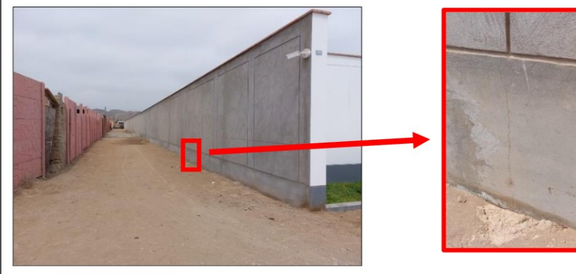
Imagen n.º 4 Fisuras verticales en el sobrecimiento de cerco perimétrico ubicado en el pasaje S/N
