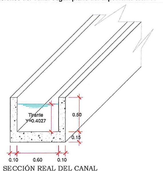
Imagen 11 Dimensiones del Canal según plano del expediente técnico
