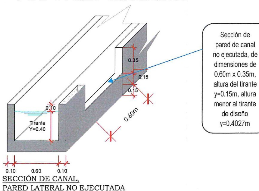
Imagen 12 Sección de pared de canal no ejecutada, progresiva 0+155 km
