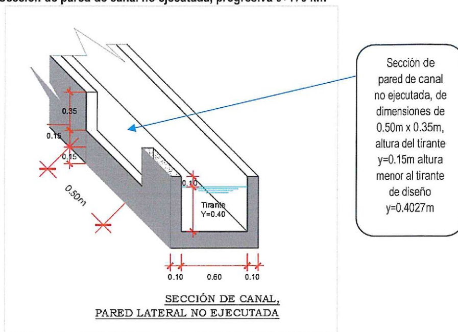
Imagen 13 Sección de pared de canal no ejecutada, progresiva 0+170 km
