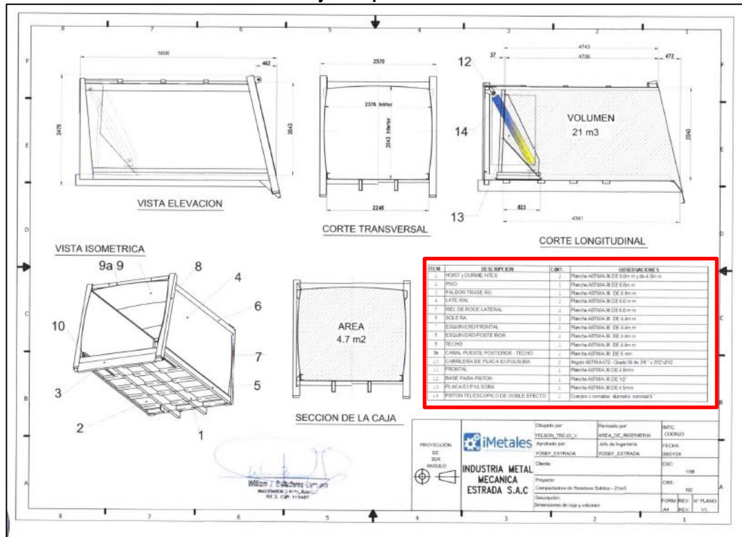
Imagen n.º 4 Plano de la caja compactadora
