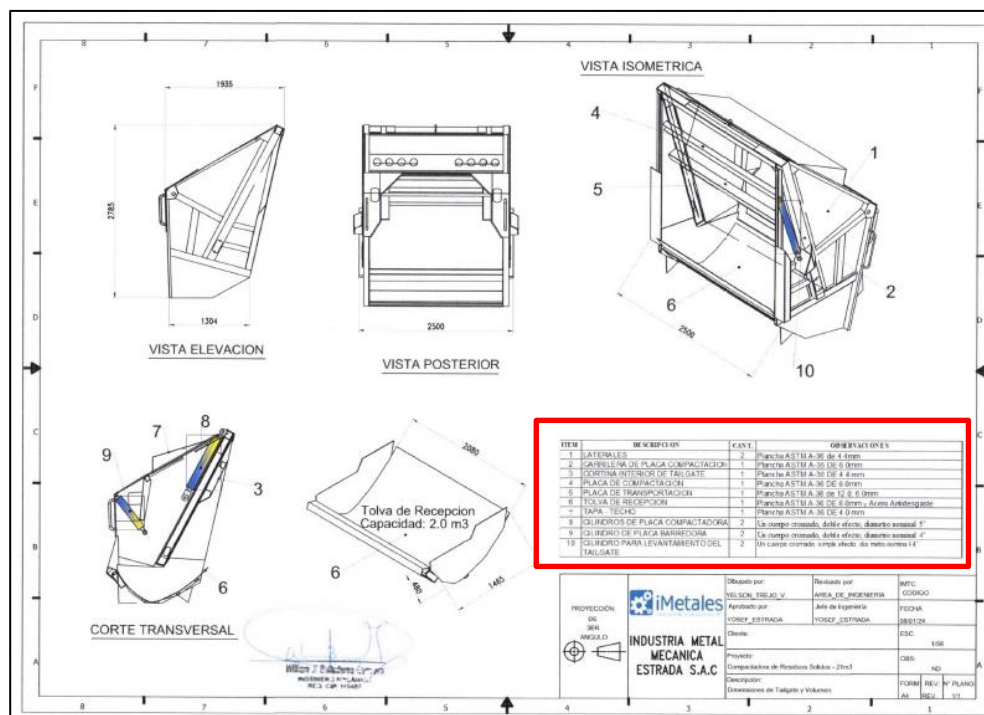
Imagen n.º 6 Plano del Tailgate
