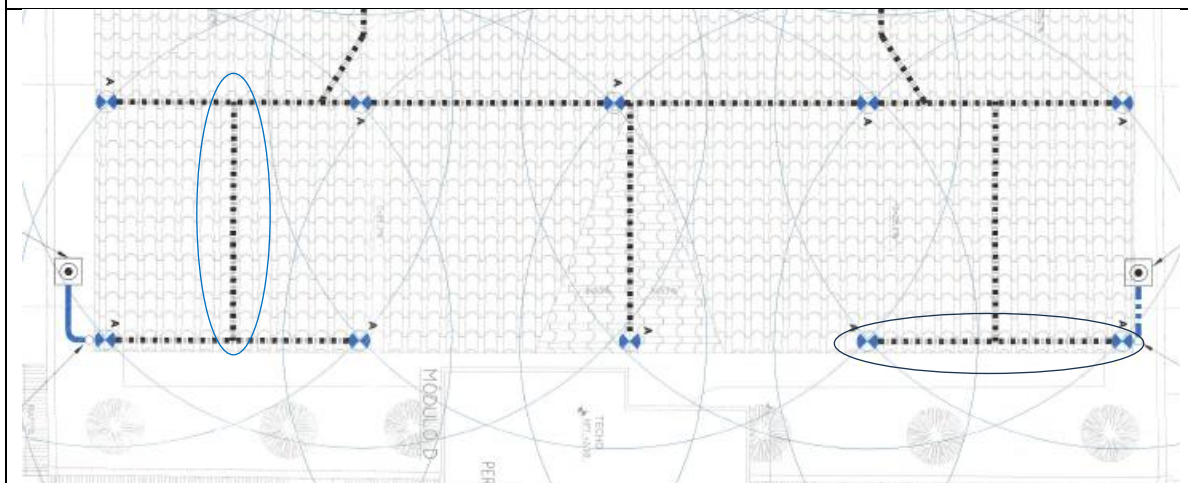
IMAGEN N° 3 PLANO SISTEMA DE PROTECCIÓN ATMOSFÉRICA LÁMINA IE-15 DE INSTALACIONES ELÉCTRICAS
