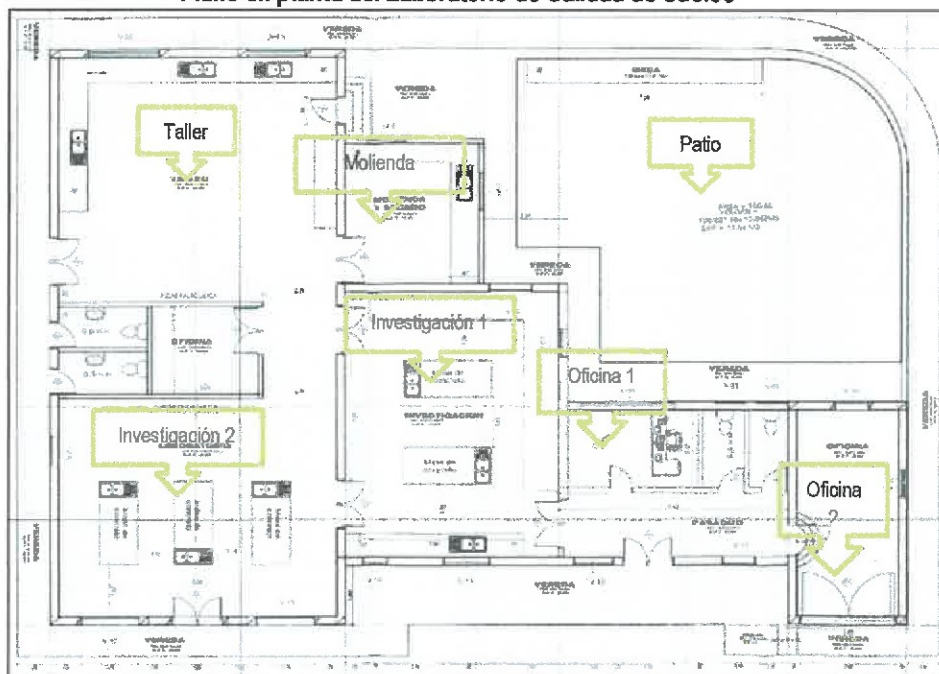
Imagen n.º 15 Plano en planta del Laboratorio de Calidad de Suelos
