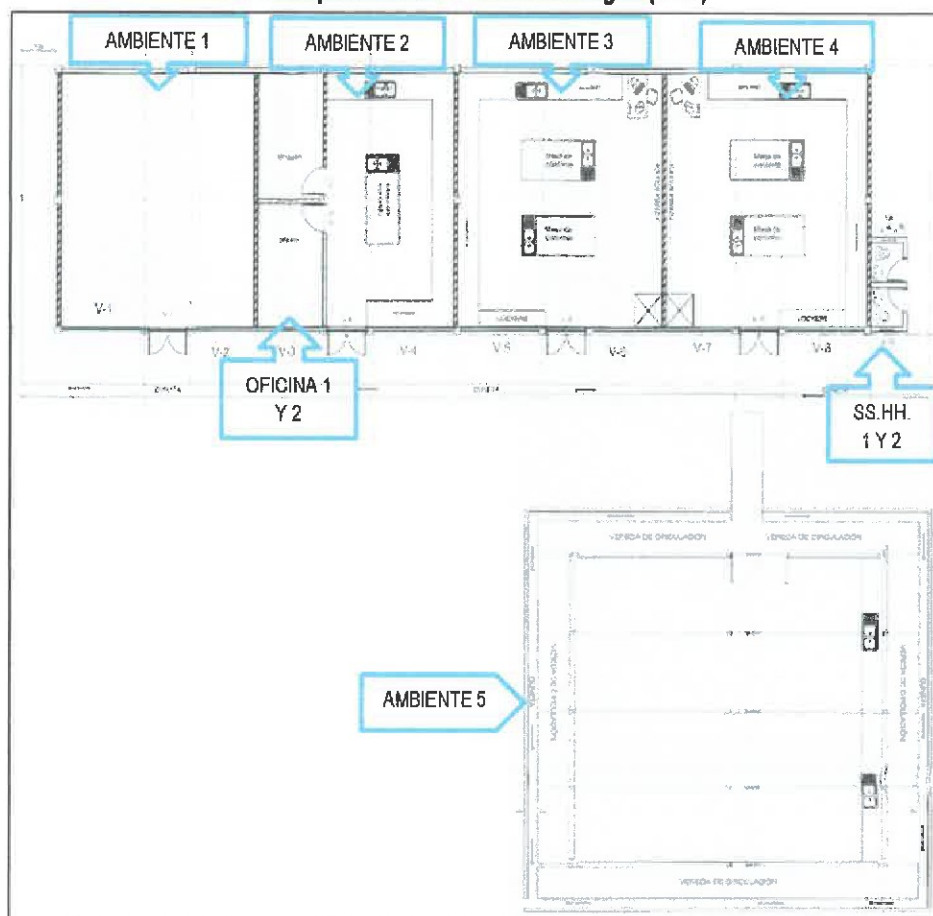
Imagen n.º 14 Plano de planta del Laboratorio de Agua (LAB)
