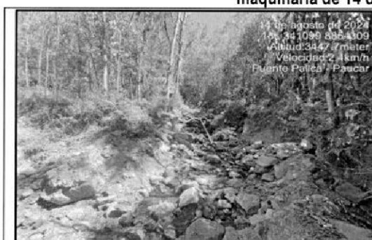
Fotografía n.º 23: En la siguiente imagen se puede visualizar el cause río arriba del puente progresiva 00+015 metros, en el que se encuentra con presencia de sedimentos y agregados grueso (piedra grande) y materia orgánica (troncos)
