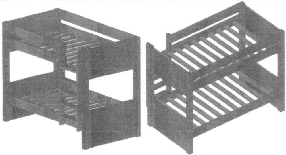
Cuadro n.º 18 Medidas e isometría de los camarotes de madera
