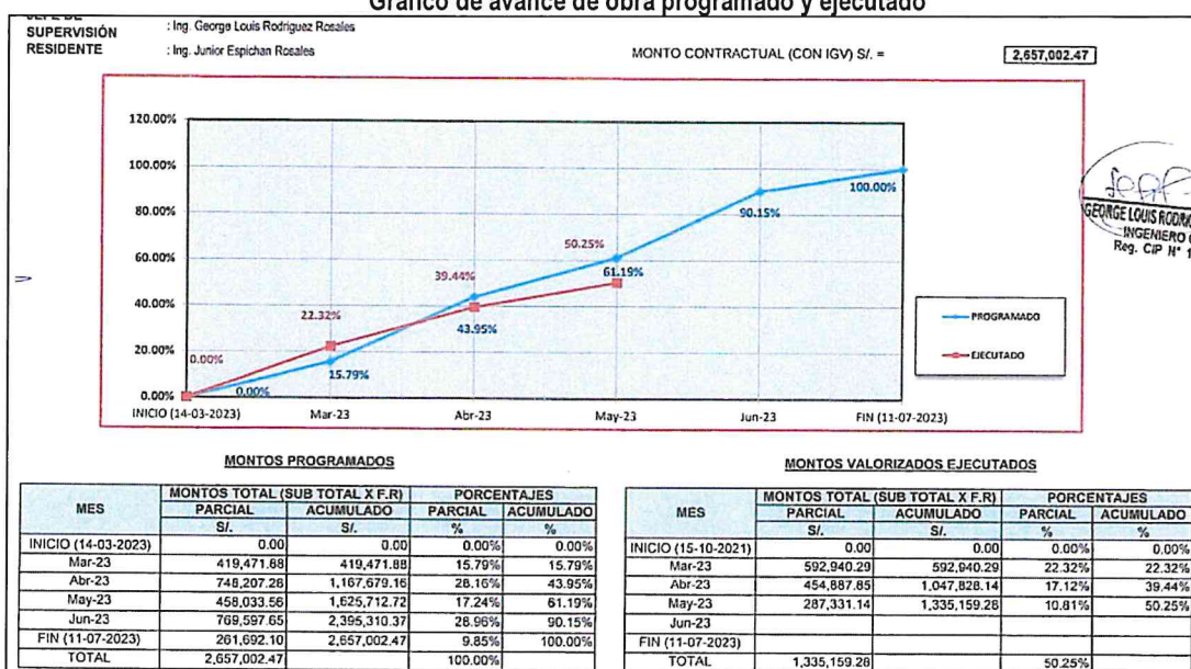
Imagen n.º 1 Gráfico de avance de obra programado y ejecutado
