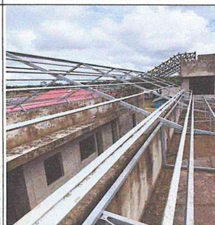
Fotografía n.º 16: En la vista se observó la inyección de cobertura y cumbrera en ambientes administrativos, ingreso principal y techo hall.
