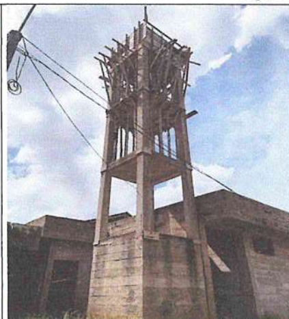
Fotografía n.º 12: En la vista se observó la inyección de desencofrado y curado en los muros laterales y losa inferior del tanque elevado.
