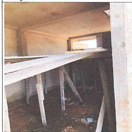
Fotografía n.º 25: En la visita se observó la inyección de falso piso y contrapiso en el ambiente de almacén.
