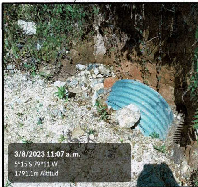
Imagen n.º 18 Alcantarilla TMC Ø 36" aplastado y colmatado Tramo: Bajo Ihuamaca – La Estrella
