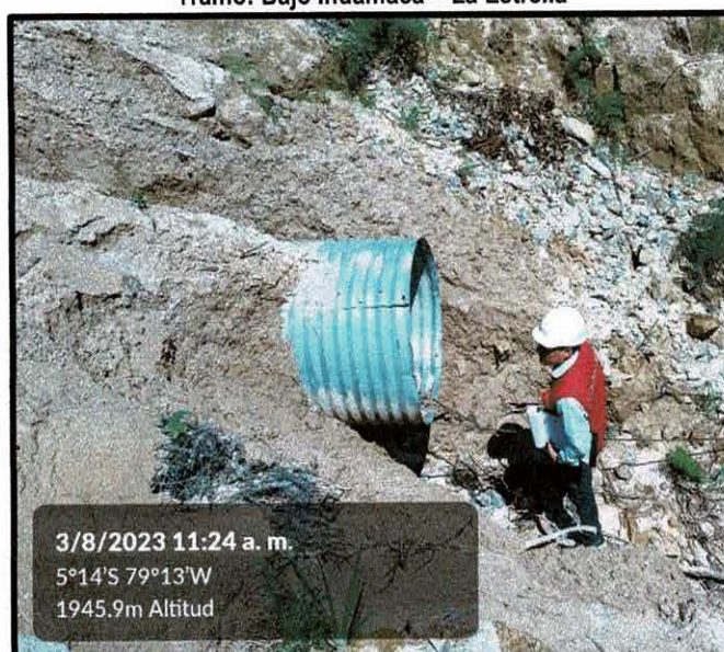
Imagen n.º 17 Alcantarilla TMC Ø 36" a la intemperie Tramo: Bajo Ihuamaca – La Estrella
