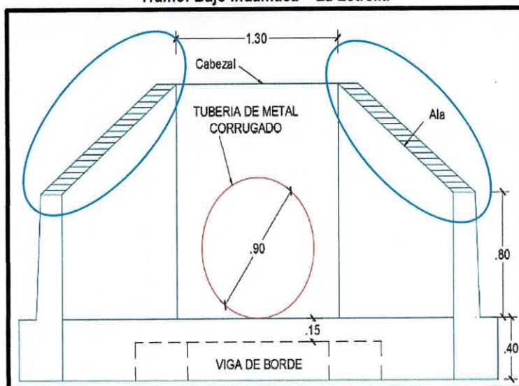
Imagen n.º 13 Aleta de concreto del cabezal – Expediente Técnico Tramo: Bajo Ihuamaca – La Estrella
