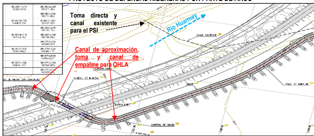
FIGURA 3. UBICACIÓN DE CANAL EXISTENTE Y ESTRUCTURAS HIDRÁULICAS DE CAPTACIÓN DEL PROYECTO DE DEFENSAS RIBEREÑAS POR PARTE DE ARCC
