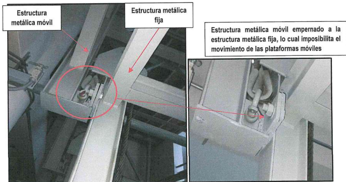
IMAGEN N° 13 PLATAFORMAS MÓVILES EMPERNADAS IMPOSIBILITANDO SU MOVIMIENTO
