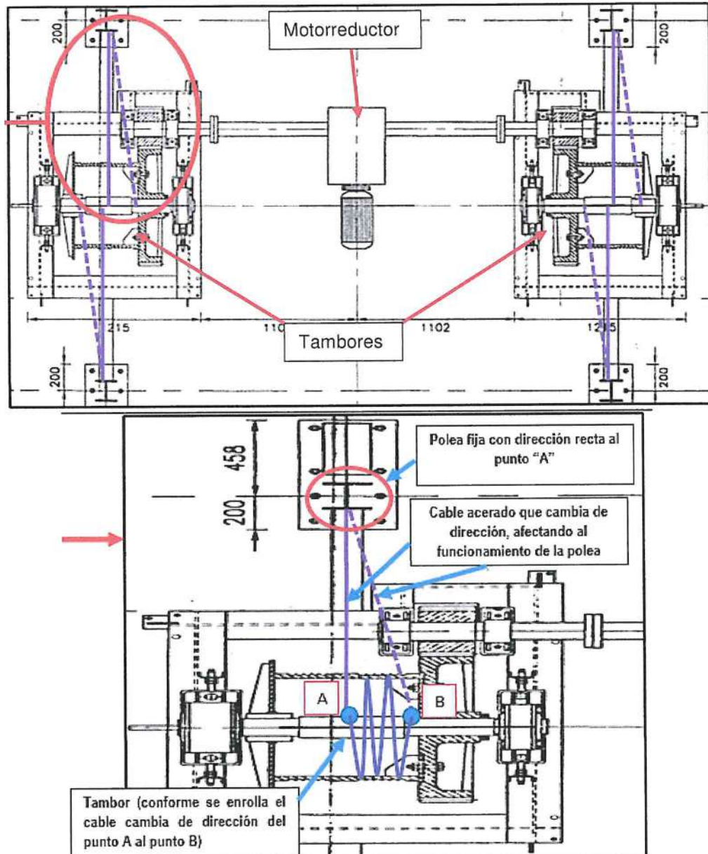
IMAGEN N° 7 DETALLE DEL GIRO DEL CABLE EN EL TAMBOR VS POLEA
