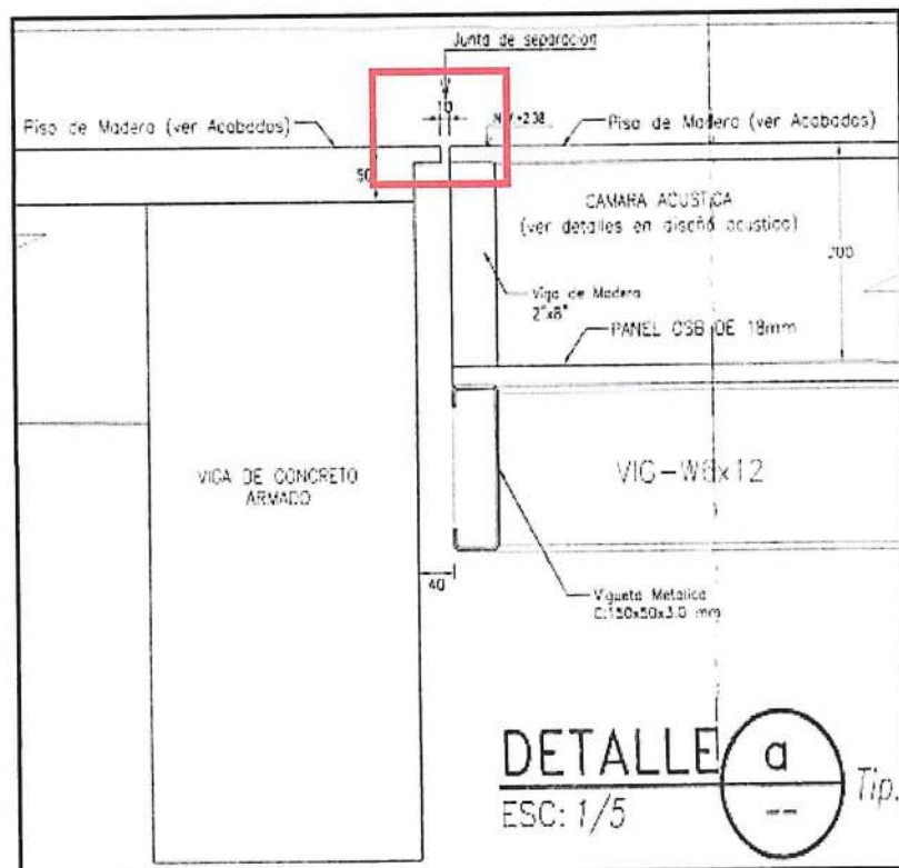
IMAGEN N° 5 DETALLE DE JUNTA DE 10MM ENTRE PLATAFORMA MÓVIL Y VIGA DE CONCRETO; Y ENTRE PLATAFORMAS MÓVILES
