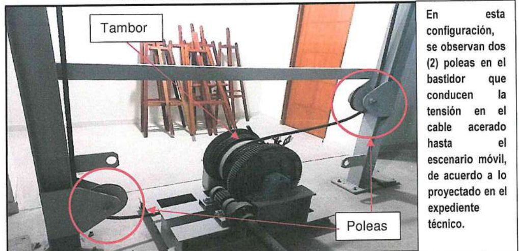
IMAGEN N° 15 DETALLE DE INSTALACIÓN DE TAMBOR Y POLEAS
