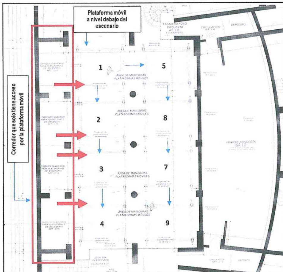
IMAGEN N° 10 VISTA DE CORREDOR CON ACCESO SOLO POR LA PLATAFORMA MÓVIL
