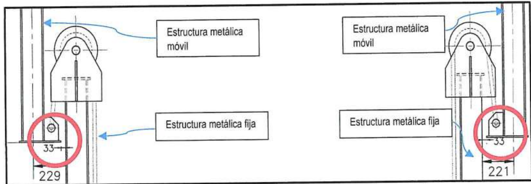
IMAGEN N° 4 DISTANCIA HORIZONTAL ENTRE LA ESTRUCTURA METÁLICA FIJA Y MÓVIL
