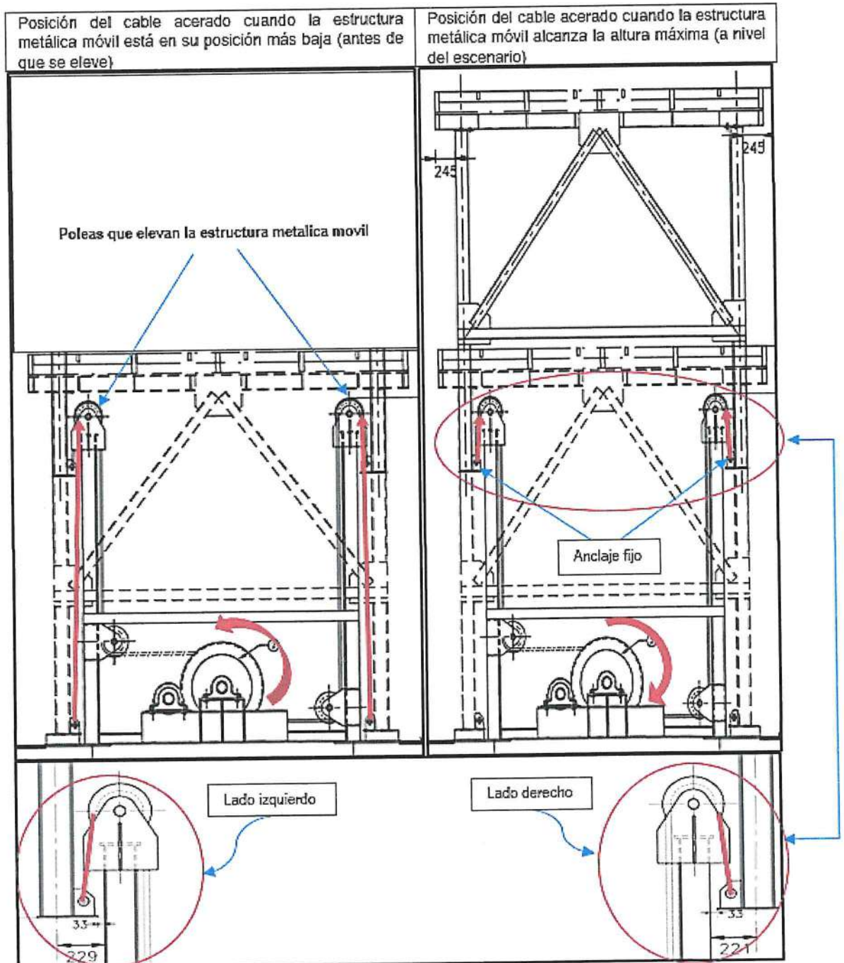
IMAGEN N° 3 ANÁLISIS DEL CABLE ACERADO ENTRE LA POLEA QUE ELEVA LA ESTRUCTURA METÁLICA MÓVIL Y EL ANCLAJE FIJO
