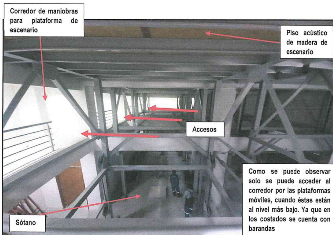
IMAGEN N° 17 VISTA DEL CORREDOR CON ÚNICO ACCESO MEDIANTE LAS PLATAFORMAS MÓVILES
