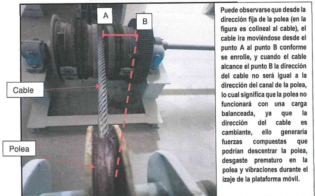
IMAGEN N° 16 DETALLE DE GIRO DE TAMBOR VS POLEA
