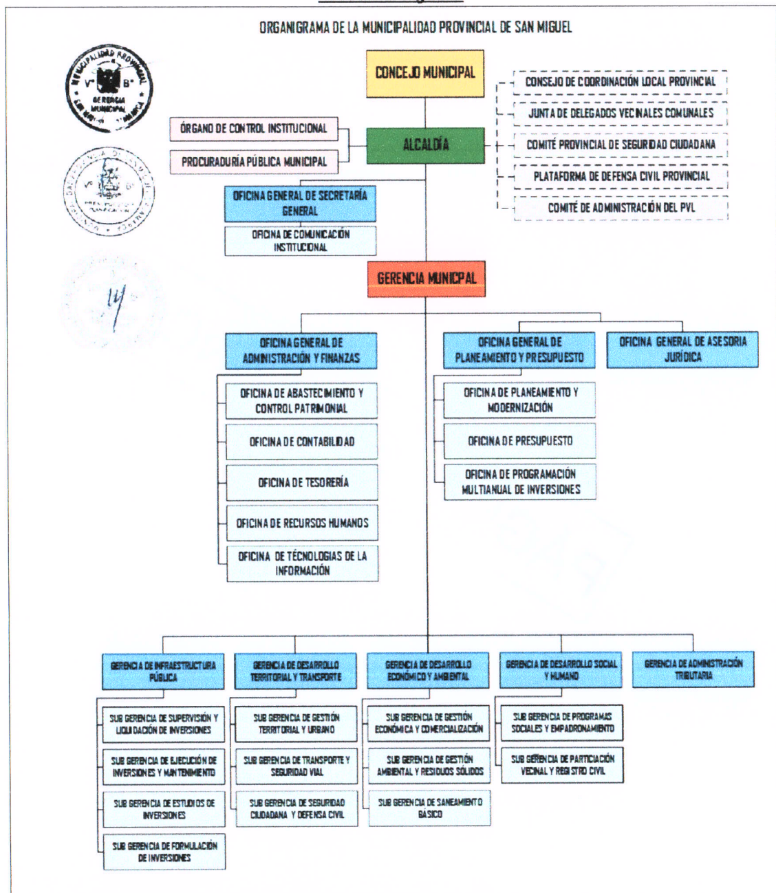
Gráfico n° 1 Estructura Orgánica
