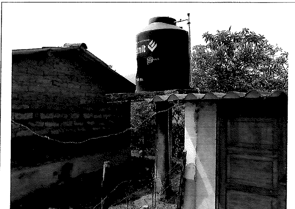
Imagen n.º 3: - La losa de estructura de concreto donde está el tanque elevado tiene rajaduras.
