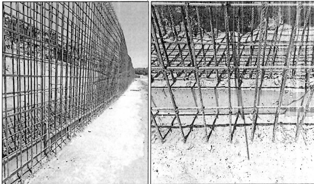
Imagen n.º 3 Fierros del muro de contención margen derecha (aguas abajo), progresivas 32+580 hasta la 32+800 con presencia de óxido
