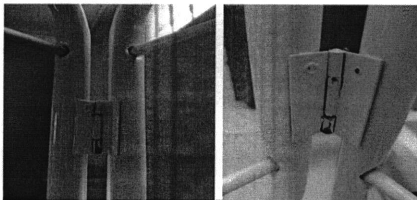
IMAGEN N°3 BISAGRAS DE LOS BIOMBOS PRESENTAN ÓXIDOS Y DESPRENDIMIENTO DE PINTURA
