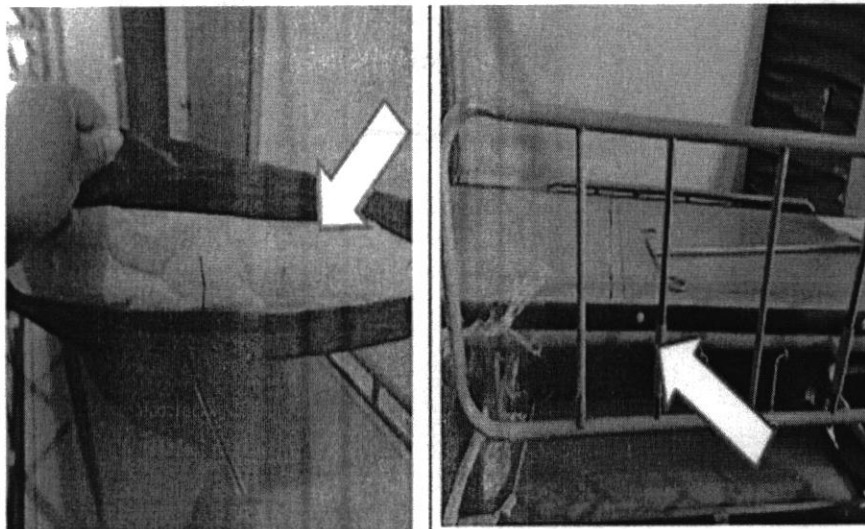
IMAGEN N°11 LA COLCHONETA ES DELGADA Y DE MATERIAL SIMPLE, CAMILLA CON BARANDAS INESTABLES, CAMILLA NO RESISTENTE PARA SOPORTAR A UNA PERSONA DE MUCHO PESO
