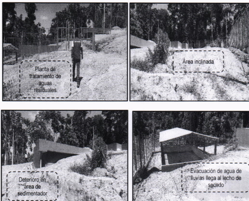
Imagen n.º 6, 7, 8 y 9 Planta de Tratamiento de Aguas Residuales
