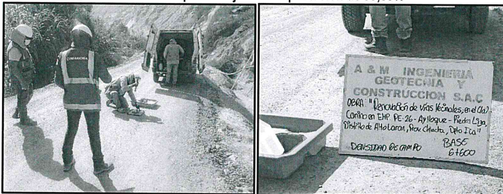
Imagen N° 1 Control de calidad de densidad en la progresiva 6+600, obteniéndose un porcentaje de compactación de 99,80%
