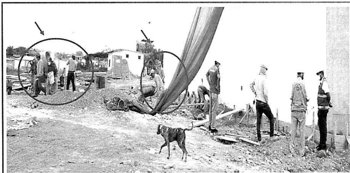
Imagen n.º 5 Personal obrero realizando trabajos sin contar con EPP
