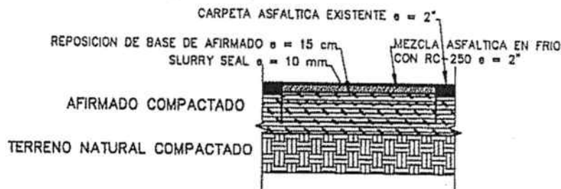
Imagen n.º 2 Espesor de Slurry Seal, según Planos del Estudio Técnico
