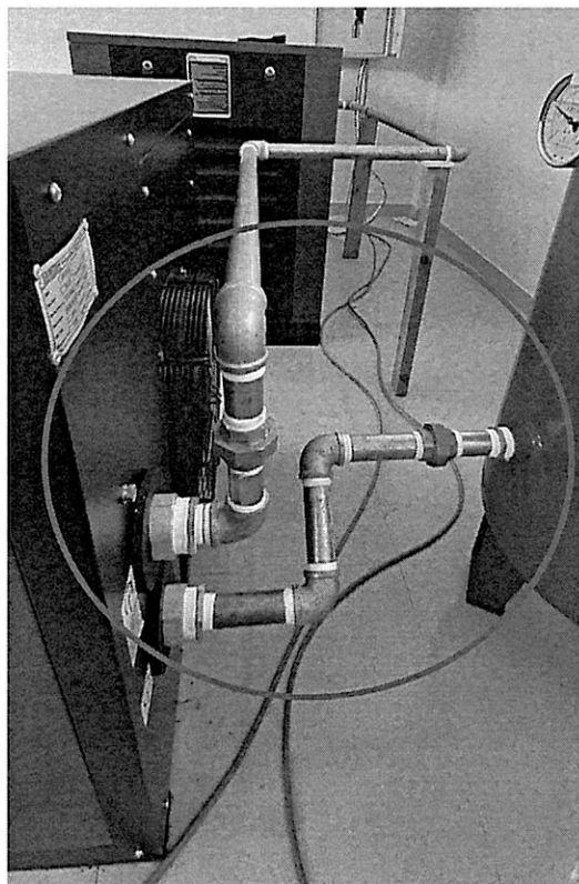
Imagen 3: Uso tubos y accesorios de fierros galvanizado, teflón (Conexión entre equipos)
