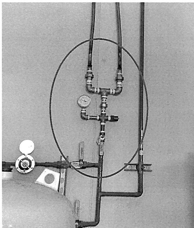
Imagen 5: Uso tubos y accesorios de fierros galvanizado, teflón (Llegada a la red de distribución Hospitalaria)
