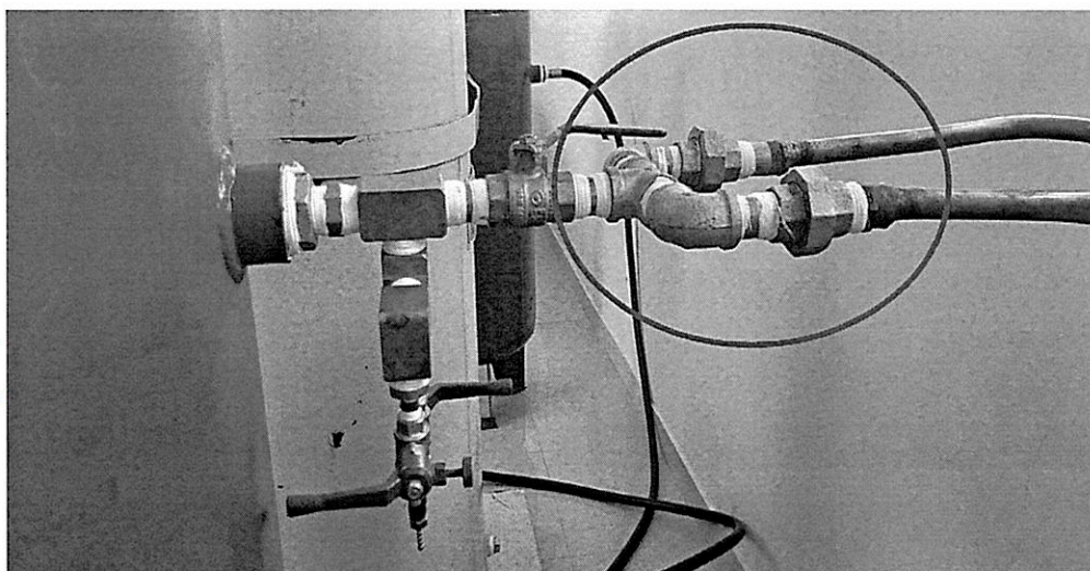
Imagen 4: Uso tubos y accesorios de fierros galvanizado, teflón (Salida desde Planta contratada)
