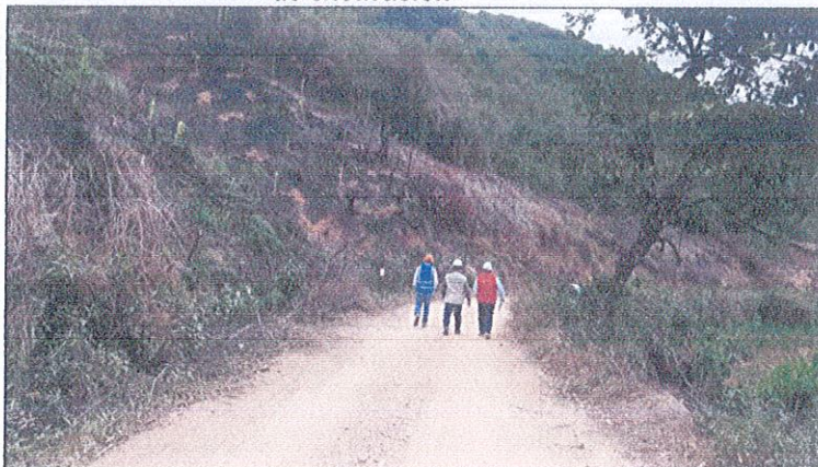
Imagen n.º 2 Tramo entre progresivas 7+585 a 8+300, no se observa trabajos de excavación
