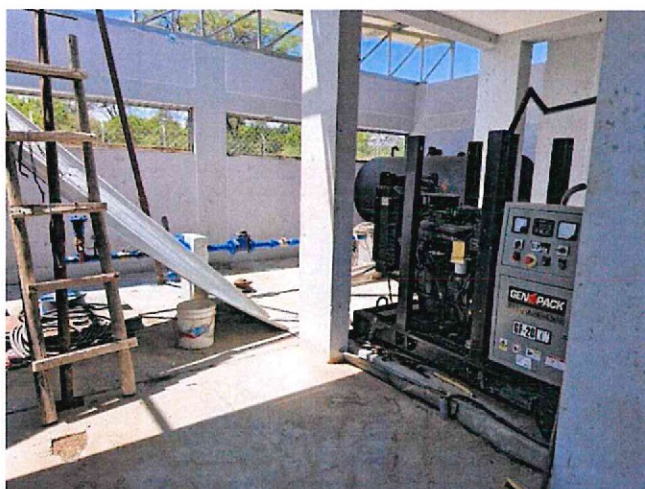
Fotografía n.º4.- Se visualiza interior de la caseta: grupo electrógeno y tuberías de impulsión.
