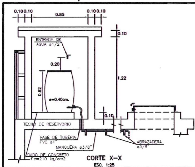
Imagen n.º 2 Plano TQ-SC-01 "Tanque elevado – Sistema de cloración"
