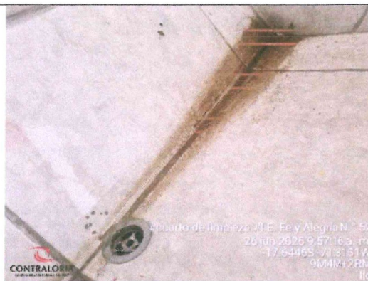
Imagen n.° 31: Defecto constructivo de pendiente.
