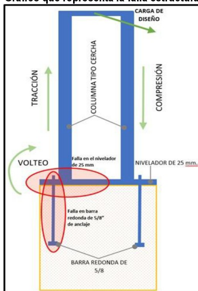
Imágenes n.º 17 Gráfico que representa la falla estructural
