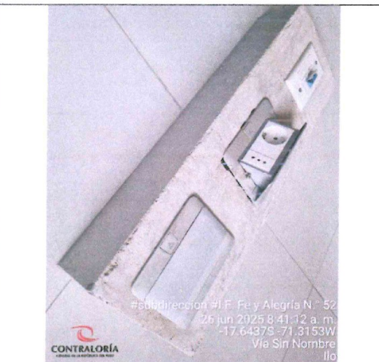
Imagen n.° 20: Toma de corriente descolocado
