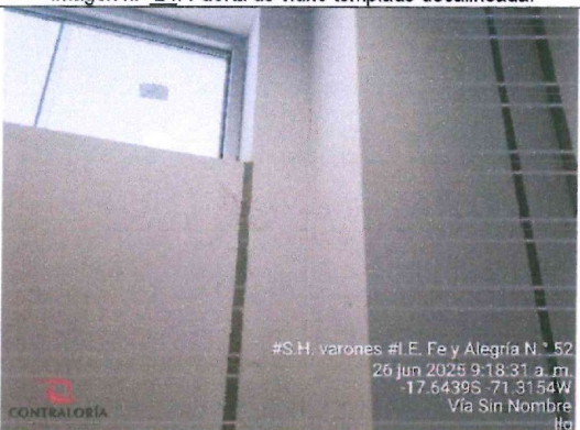
Imagen n.º 26: Fisura en unión muro-columna.
