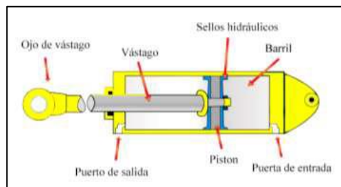
Imagen n.º 6 Esquema de un cilindro hidráulico
